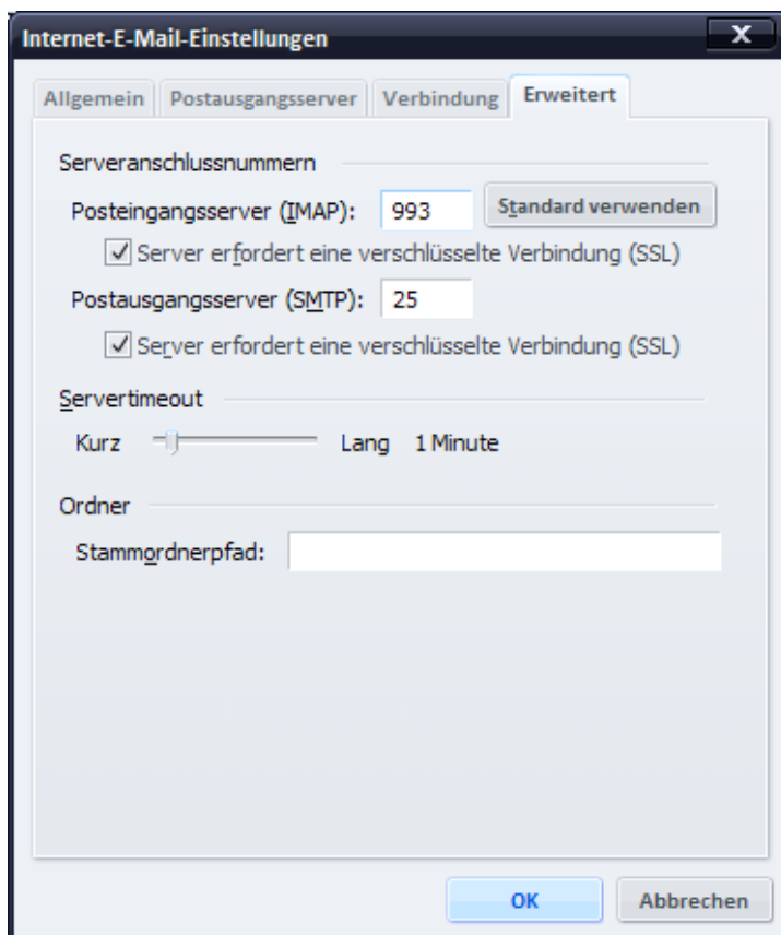
Abb. 6: Aktivieren Sie die verschlüsselte Verbindung für beide Server und klicken Sie OK.
